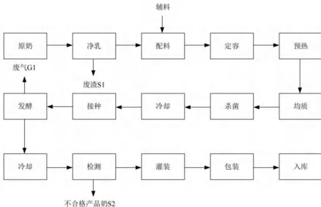
图 2-2 酸奶生产工艺流程与产污环节示意图
