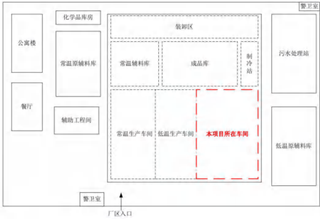
附图 3-1 厂区平面布置示意图
